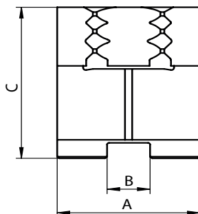
* 1 SATZ BACKEN (3 STÜCK) * SET OF 3 JAWS
